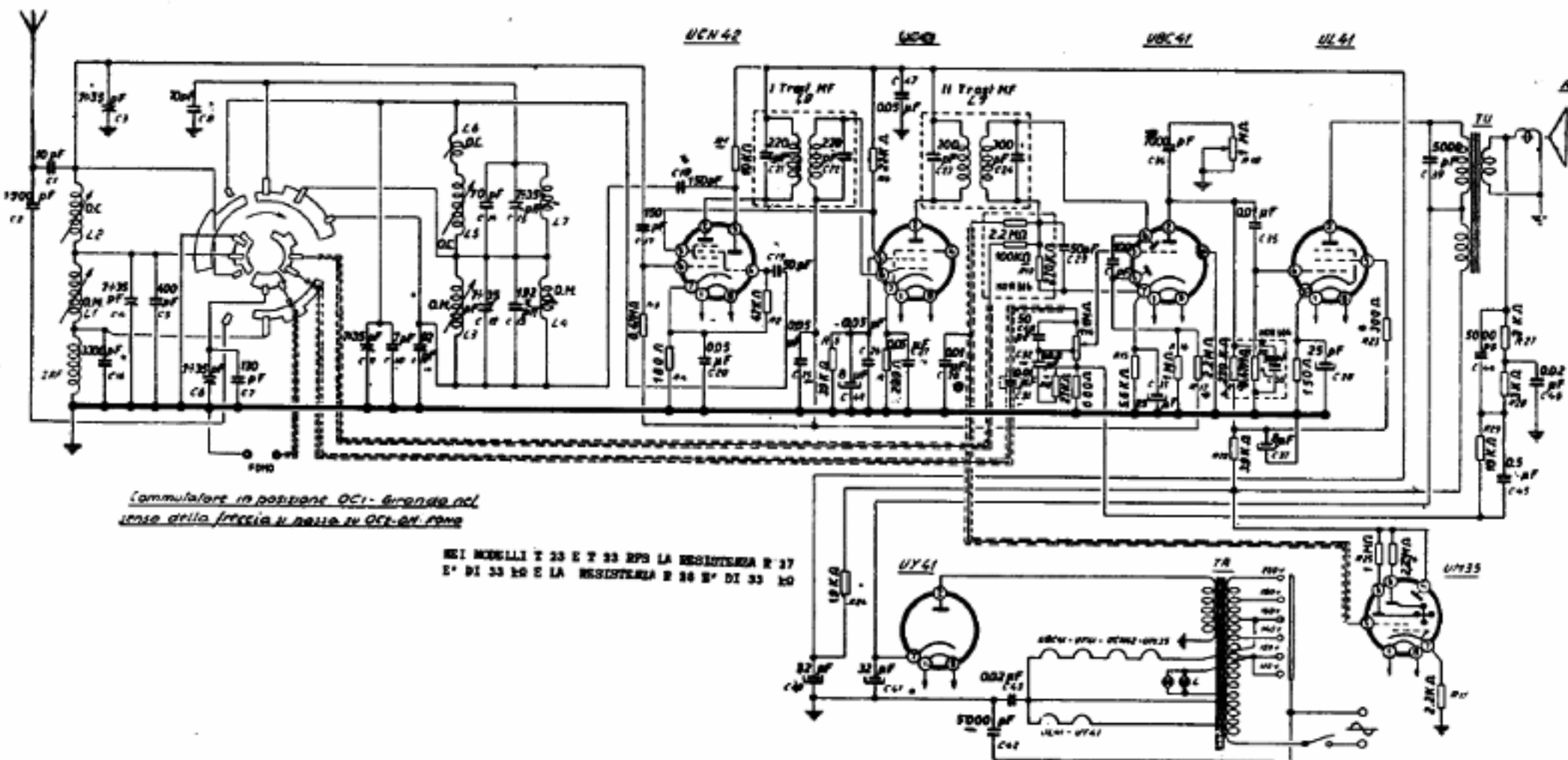
TELEFUNKEN (COMPAGNIA RADIORICEVITORI) - Modd. T 33/B, T 23 e T 23 RFS. Media frequenza 468 kc/s. Gamme di ricezione 3: OM: 185-580 m; OC1: 16-35 m; OC2: 35-78 m. Tens. anodica al primo condensatore elettrolitico: 235 V, al secondo: 185 V. Potenza d'uscita con 10 per cento di distorsione watt 3,2. Consumo watt 44.
